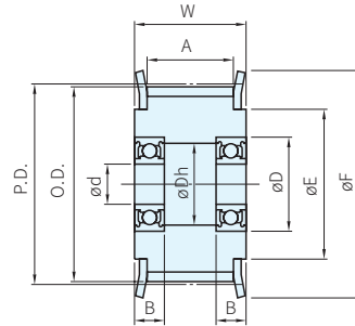
兩端軸承型 WWBKA TWBKA NWBKA
