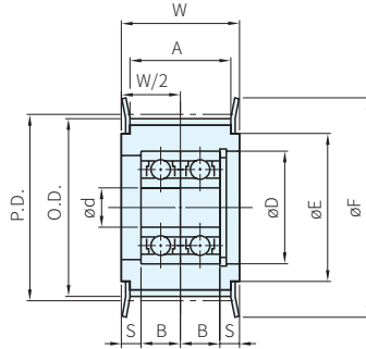
中心軸承型 (2PCS軸承時) WWBK TWBK NWBK
